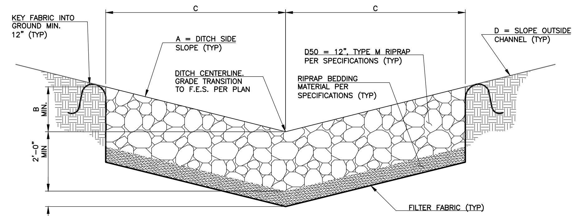
B RIPRAP SECTION SCALE: 1/2" = 1'-0"
