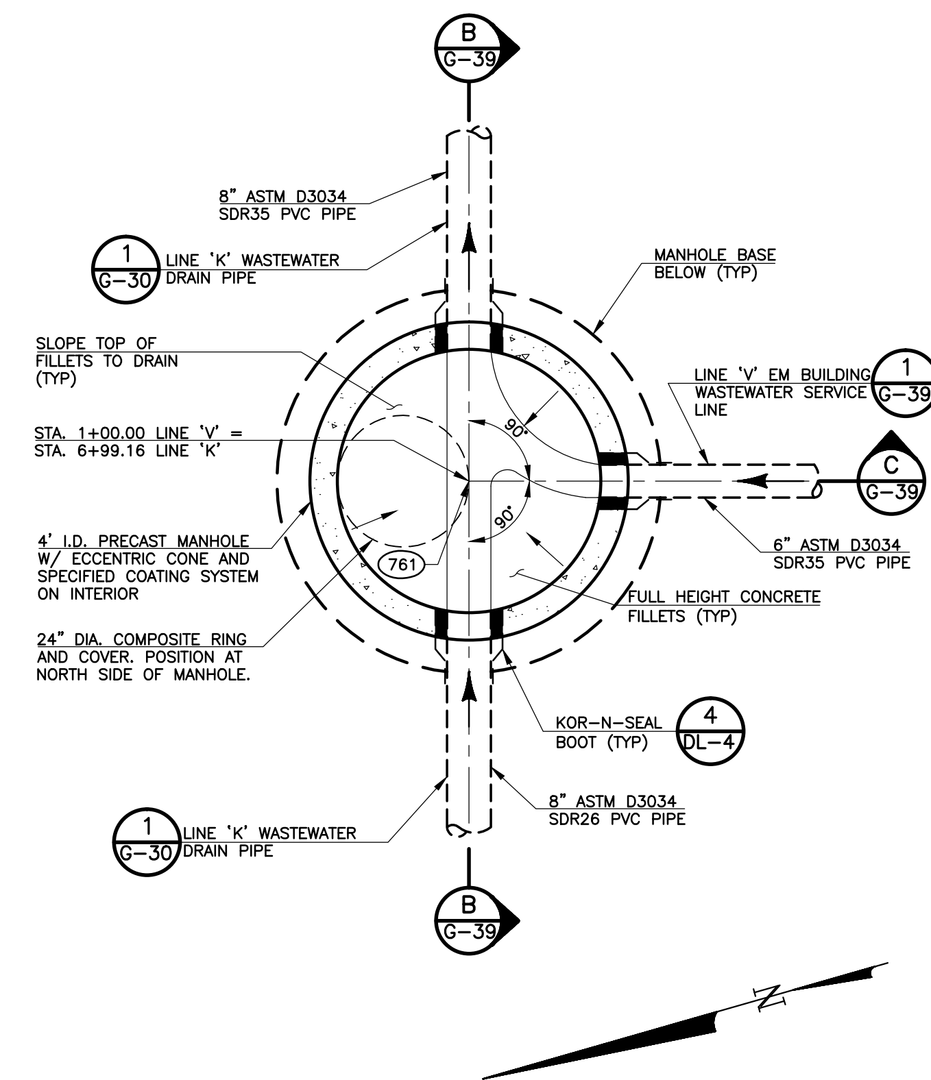
2 MANHOLE MH-12A PLAN SCALE: 1/2" = 1'-0"
