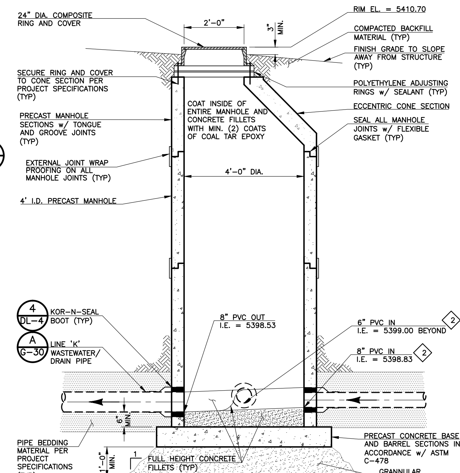
B MANHOLE MH-12A SECTION SCALE: 1/2" = 1'-0"
