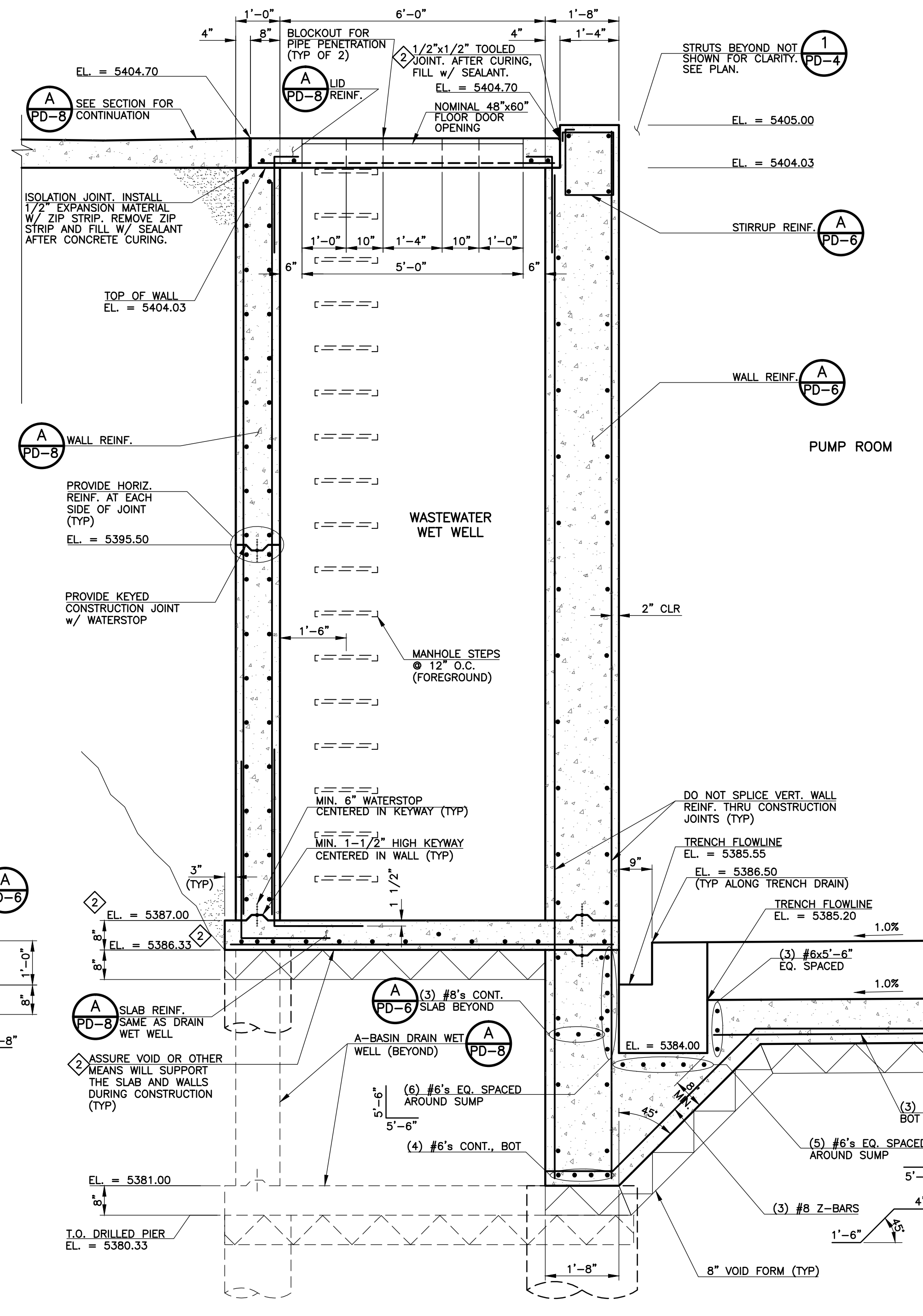
SECTION B SCALE: 1/2" = 1'-0"
