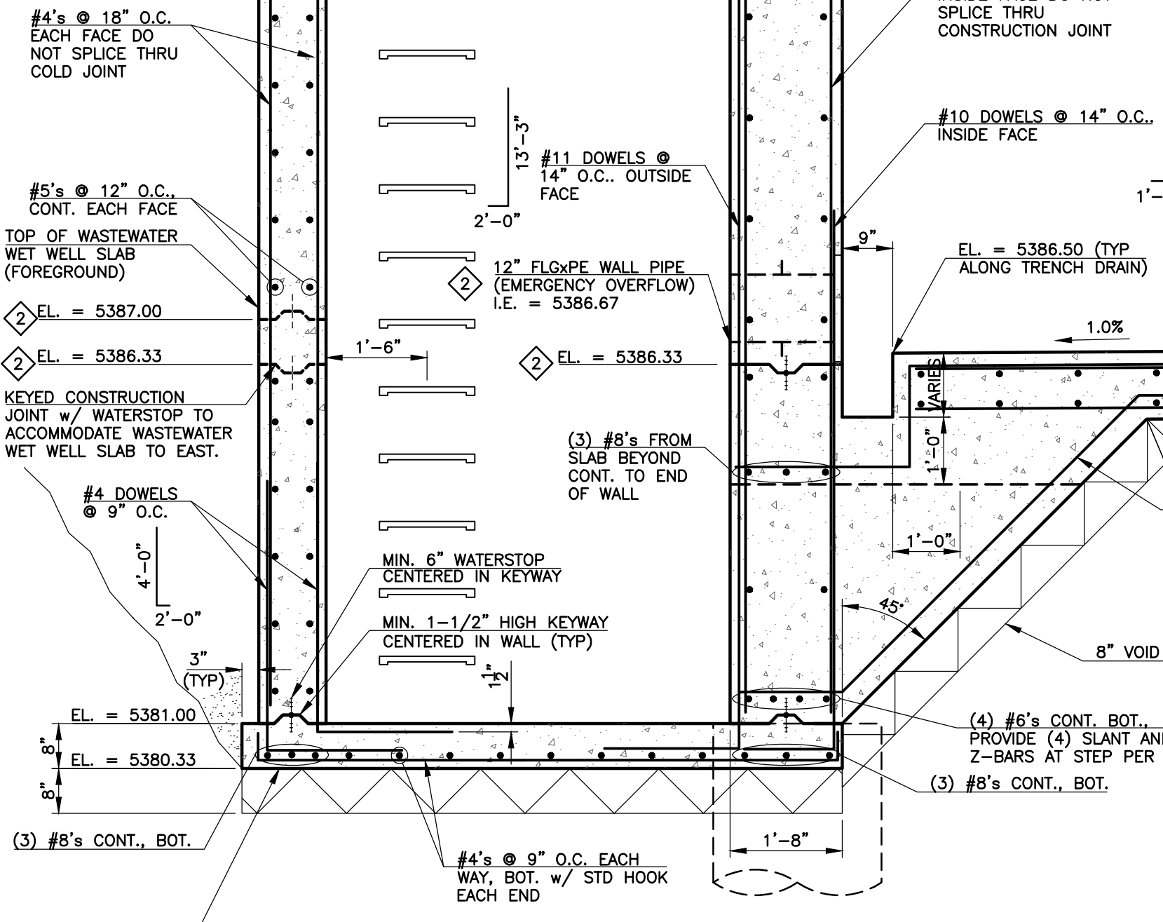
SECTION A SCALE: 1/2" = 1'-0"
