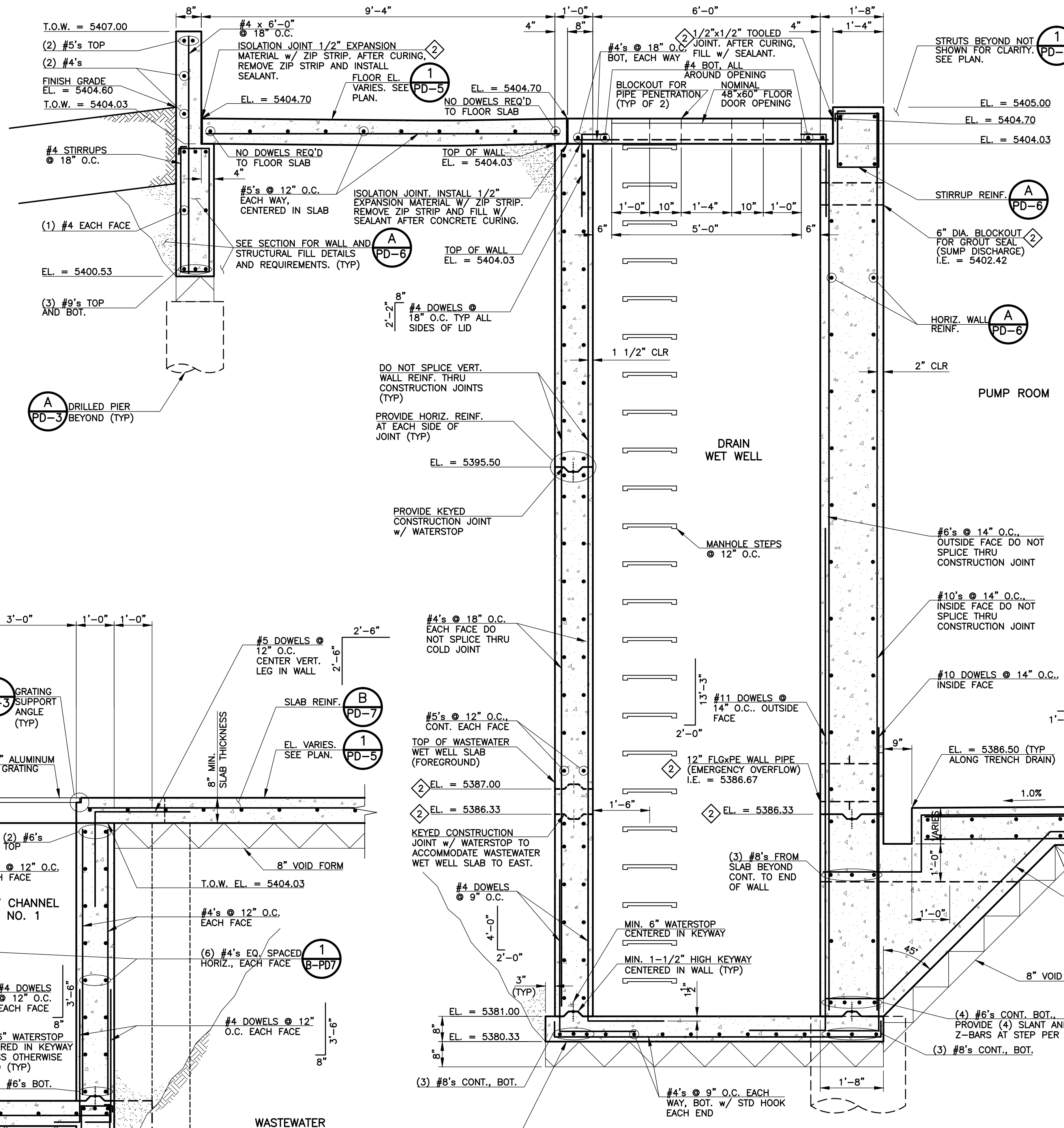
SECTION A SCALE: 1/2" = 1'-0"
